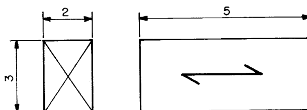
Figura B.2 - Corpo-de-prova para determinação da umidade da madeira
