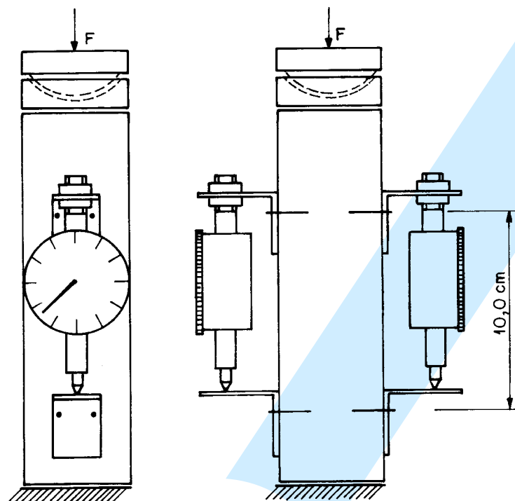
Figura B.6 - Arranjo de ensaio para compressão paralela às fibras, com instrumentação baseada em relógios comparadores
