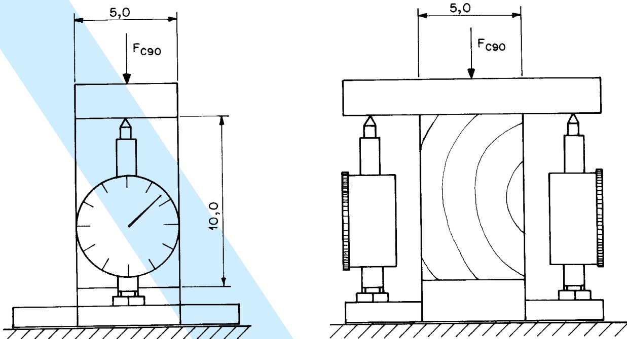
Figura B.14 - Arranjo de ensaio para compressão normal às fibras
