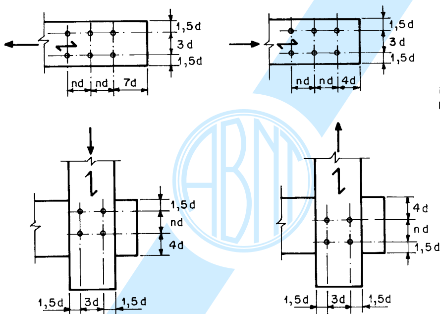
Figura 14 - Espaçamentos em ligações com pinos
