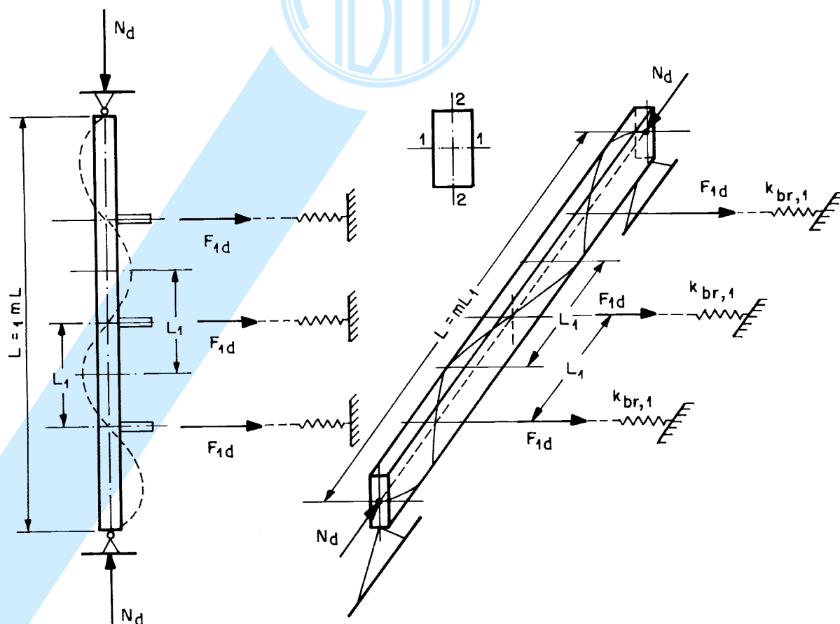
Figura 4 - Parâmetros para verificação da estabilidade lateral
