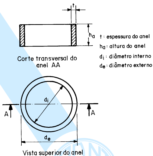
Figura C.8 - Anel metálico
