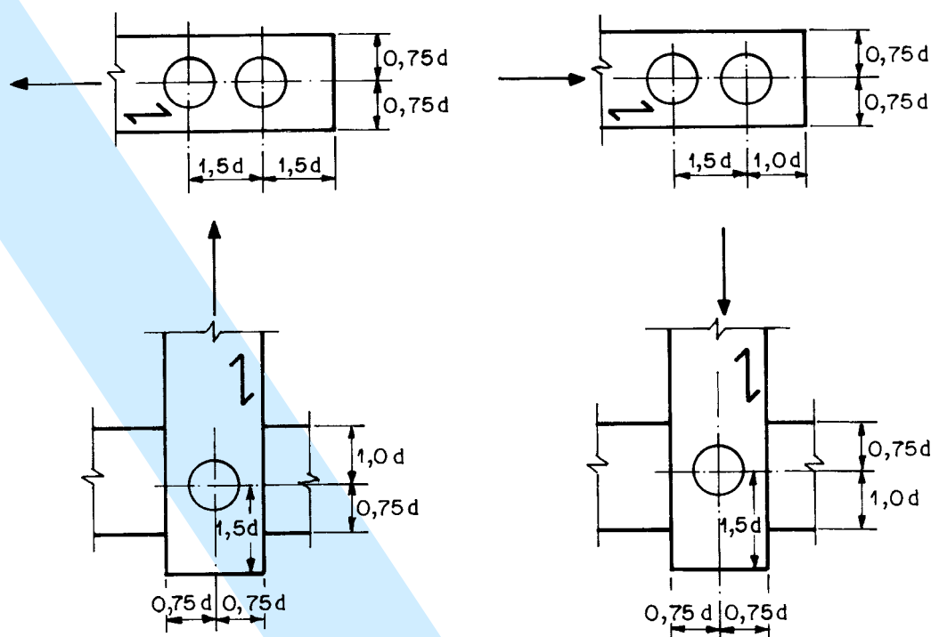
Figura 15 - Espaços em ligações com anéis metálicos
