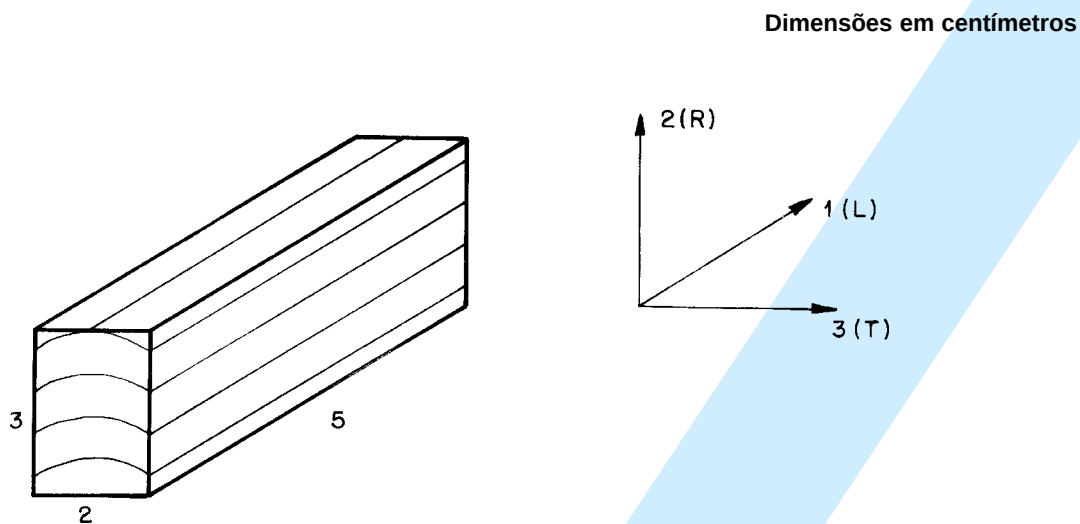
Figura B.3 - Corpo-de-prova e sistema de orientação para determinação das propriedades de retração e inchamento
