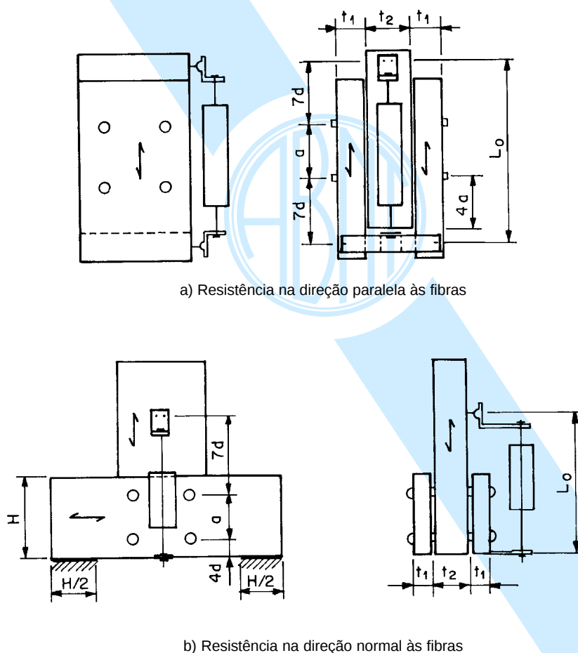
Figura C.4 - Corpos-de-prova para ensaios de ligações mecânicas
