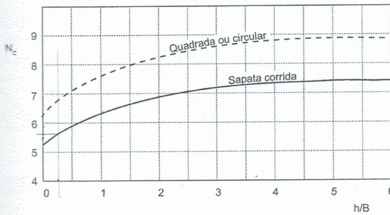
Figura 9 Fator de capacidade de carga (Skempton, 1951).
